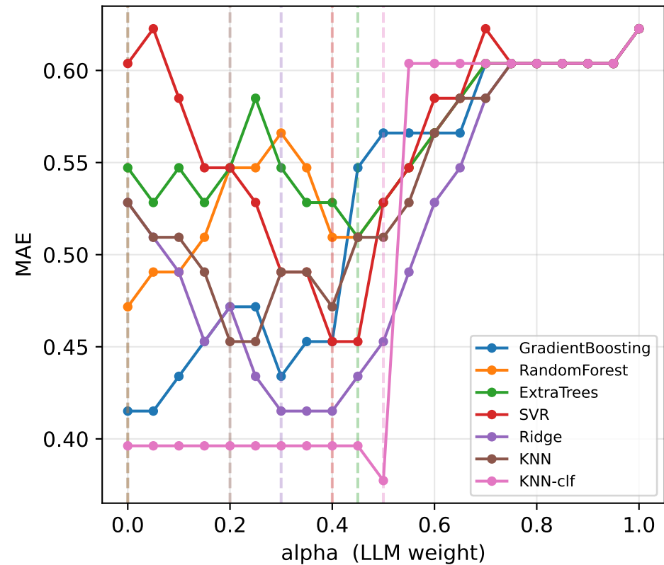
MAE
